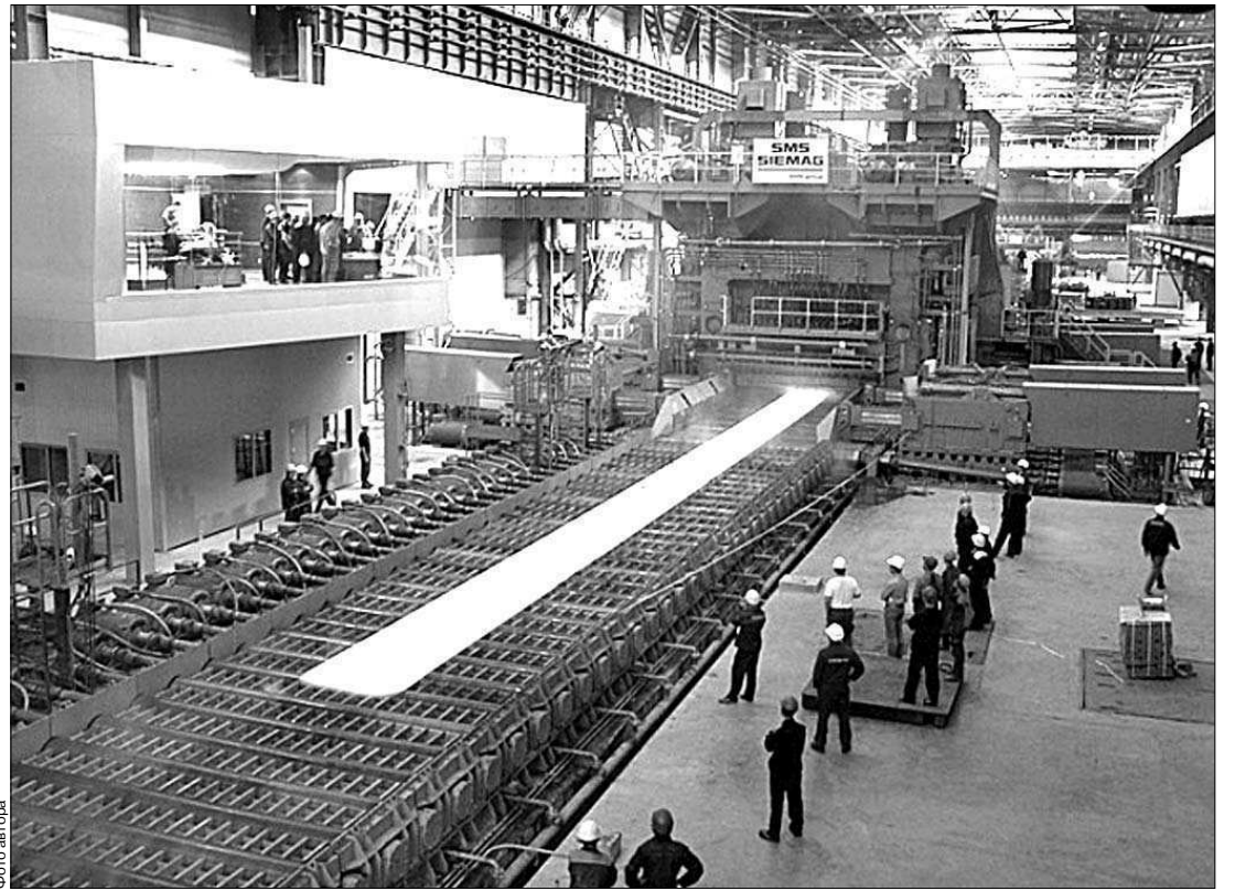
▲ Крупнейший инвестиционный проект Магнитки – стан «2000»
